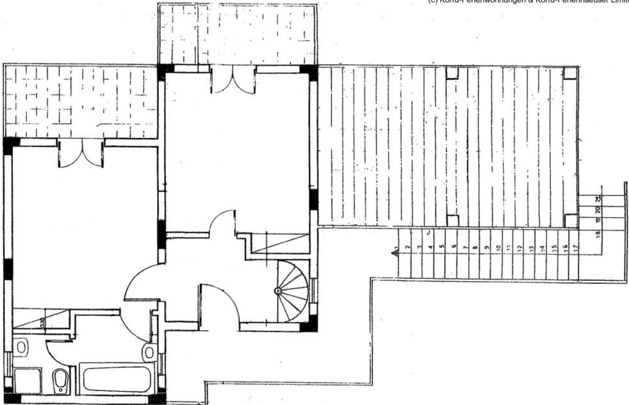
Grundriss OG Korfu - Ferienhaus Grigoris mit Privat-Pool in Agios Georgios Pagi
